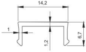
* 4112 Kapak 0,078 kg/mt
