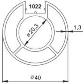
* 2246 40'lık Tek Kanal Dikme 1,3mm 0,806 kg/mt
