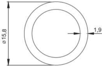
* 1234 16'lık Boru 1,9mm 0,224 kg/mt
