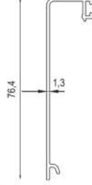
* 11495 Zemin Üstü Cam Kanal Profili 0,395 kg/mt
