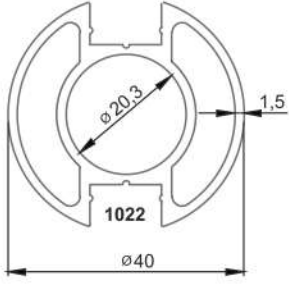
* 1565 40'lık Çift Kanallı Dikme 1,5mm 0,911 kg/mt
