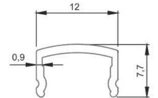
* 1022 40'lık Dikme Kapağı 0,073 kg/mt
