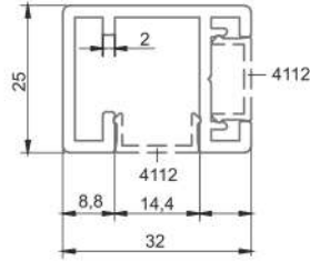
* 4105 25x32 Kare Cam Profil 0,588 kg/mt
