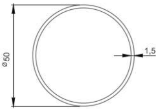
* 2622 50'lik Boru 1,5 mm 0,738 kg/mt
