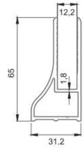
* 4891 Alt Etek Profili Tekli 1,054 kg/mt
