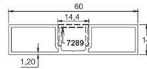
* 7277 60x14 Çit Profili 0,523 kg/mt
