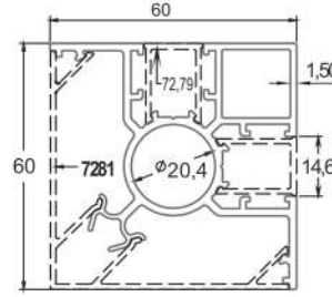
* 7272 60x60 Çit Dikme Profili 1,376 kg/mt
