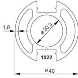
* 1010 40'lık Çift Kanallı Dikme 1,8 mm 1,143 kg/mt
