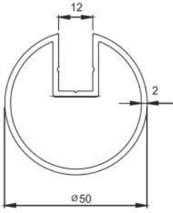
* 4723 50'lik Kanallı Profil 2mm 1,026 kg/mt
