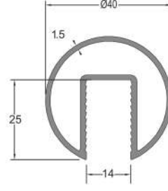
* 12150 40'lık Kanallı 14mm 0,729 kg/mt
