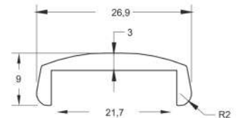
* 12281 Cam U Profili 0,234 kg/mt
