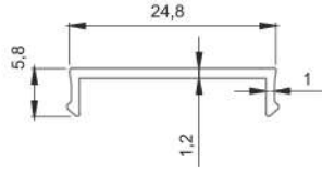
* 4113 Kapak 0,108 kg/mt
