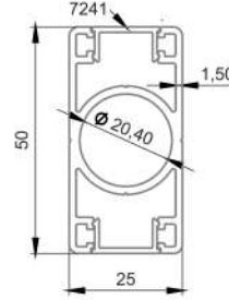
* 7252 25x50 Çift Kanallı Dikme 0,857 kg/mt
