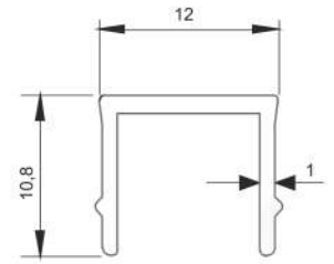
* 4099 Kapak 0,094 kg/mt
