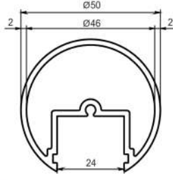
* 3809 50'lik Kanallı Boru 24mm 1,050 kg/mt
