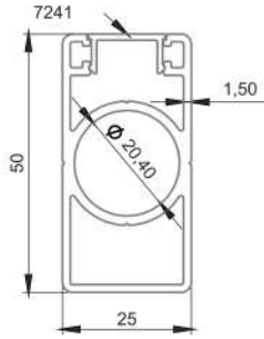
* 7253 25x50 Tek Kanallı Dikme 0,872 kg/mt
