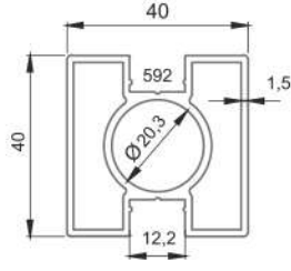
* 5434 40x40 Kare Dikme Profili (1,5mm) 1,020 kg/mt
