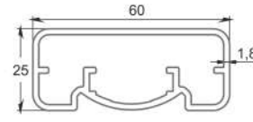
* 3627 25x60 Kare Profil Ay Bağlantılı 0,938 kg/mt
