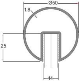
* 12152 50'lık Kanallı 14mm 1,003 kg/mt
