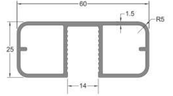
* 12154 25x60 Kare Camlı Profil 14mm 0,829 kg/mt
