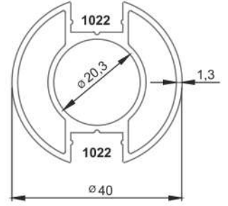
* 2879 40'lık Çift Kanal Dikme 1,3mm 0,755 kg/mt
