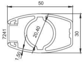
* 7804 30x50 Tek Kanal Dikme Profili 0,900 kg/mt
