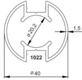
* 1599 40'lık Çift Kanal Dikme 1,5mm 0,762 kg/mt
