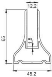
* 4892 Alt Etek Profili Çiftli 1,196 kg/mt
