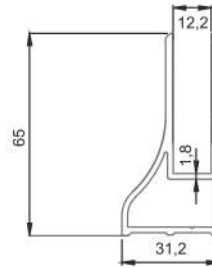
* 4891 Alt Etek Profili Tekli 1,054 kg/mt
