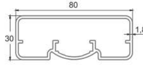
* 3631 30x80 Kare Profil 1,183 kg/mt
