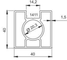
* 5678 40x40 Kare Tek Kanal Dikme Profili (1,5mm) 1,046 kg/m
