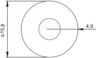
* 916 16'lık Boru 4,9mm 0,454 kg/mt
