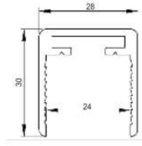
* 7311 Cam U Profili 0,528 kg/mt
