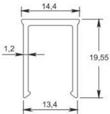
* 7279 Kapak 0,175 kg/mt
