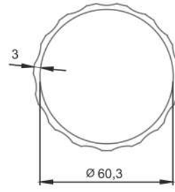
* 1036 65'lik Tırtıllı Boru 1,377 kg/mt
