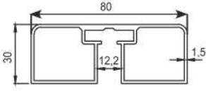
* 4894 30x80 Kare Profil 12mm 1,187 kg/mt
