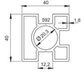
* 591 40x40 Kare Profili (1,8mm) 1,183 kg/mt
