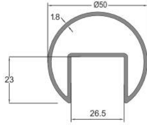
* 12153 50'lık Kanallı Boru 26,5mm 0,946 kg/mt
