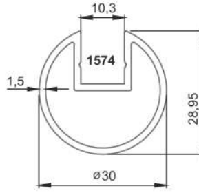
* 1570 30'luk Kanallı Profil 1,5mm 0,467 kg/mt
