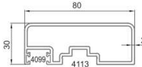
* 4761 30x80 Kare Profil 1,322 kg/mt
