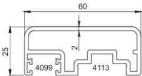
* 4096 25x60 Kare Profil 1,072 kg/mt
