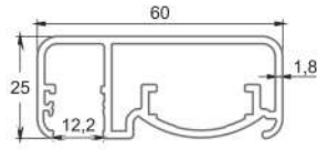
* 3626 25x60 Kare Profil Cam Kanallı 0,976 kg/mt
